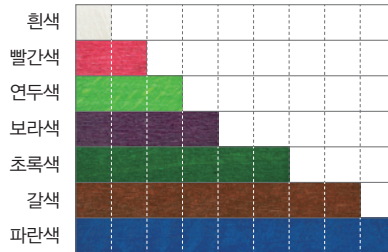
직선 모델
